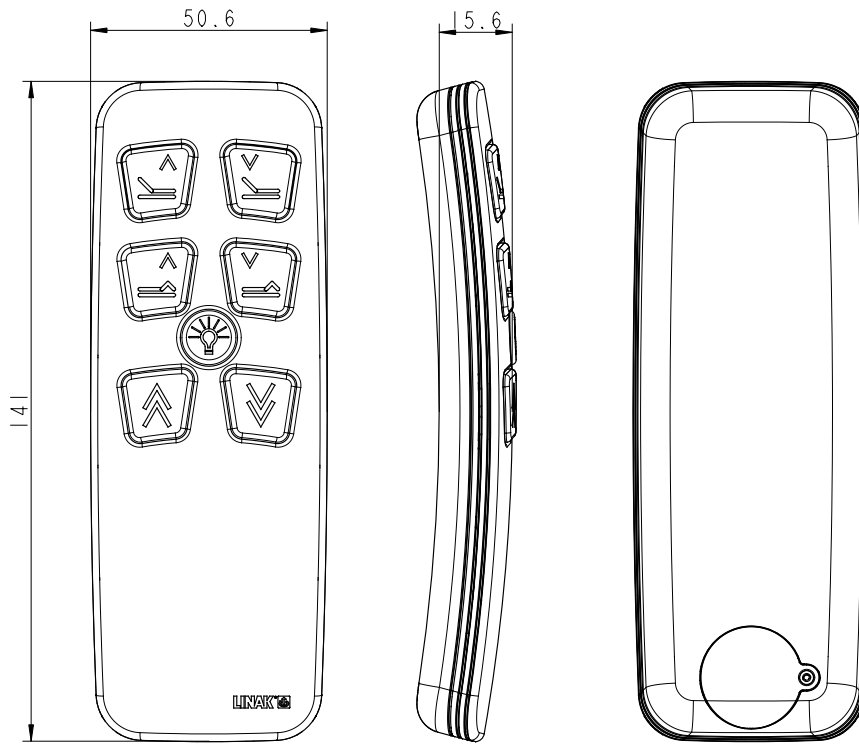
Dimensioni HC10 wireless (mm)
