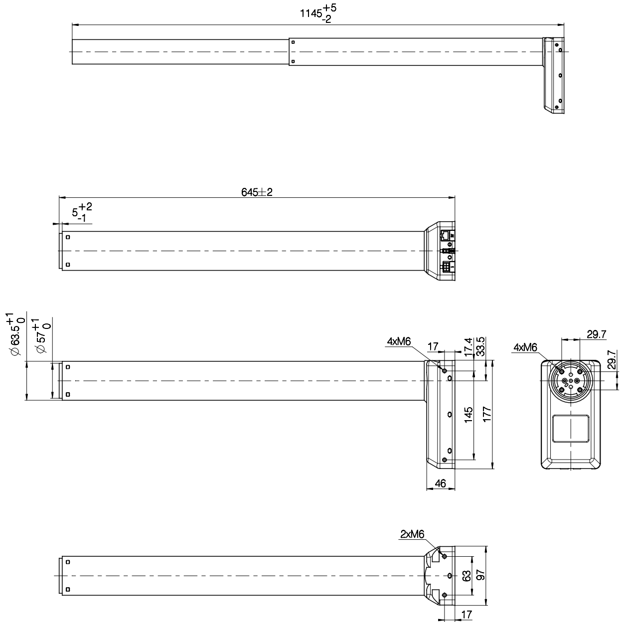
Dimensioni DL8 IC Master (mm)
