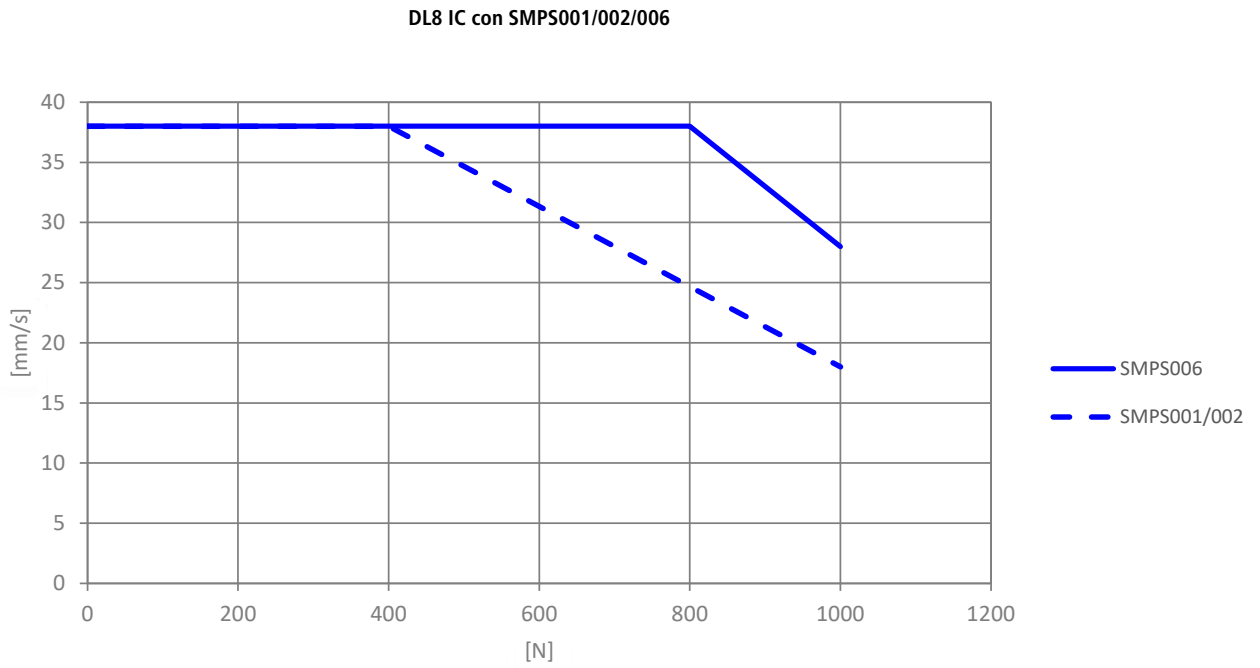
Due DL8 IC (carico uniforme) con SMPS001/002/006
