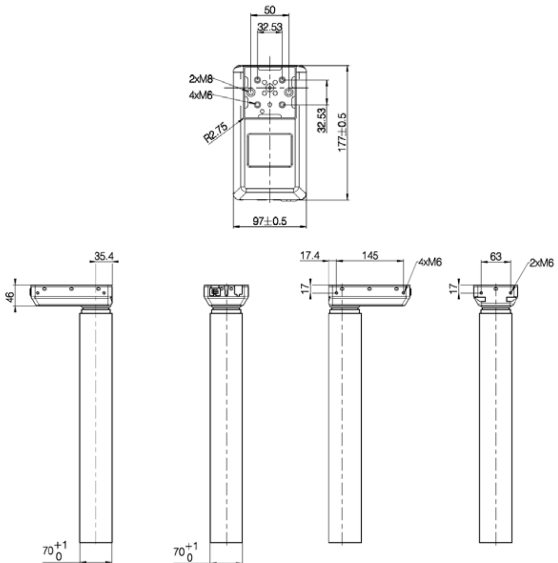
DL19 IC dimensioni scatola motore e profili (mm)
