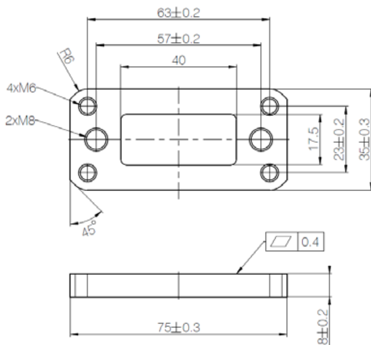
Dimensioni staffa di fissaggio (mm)
