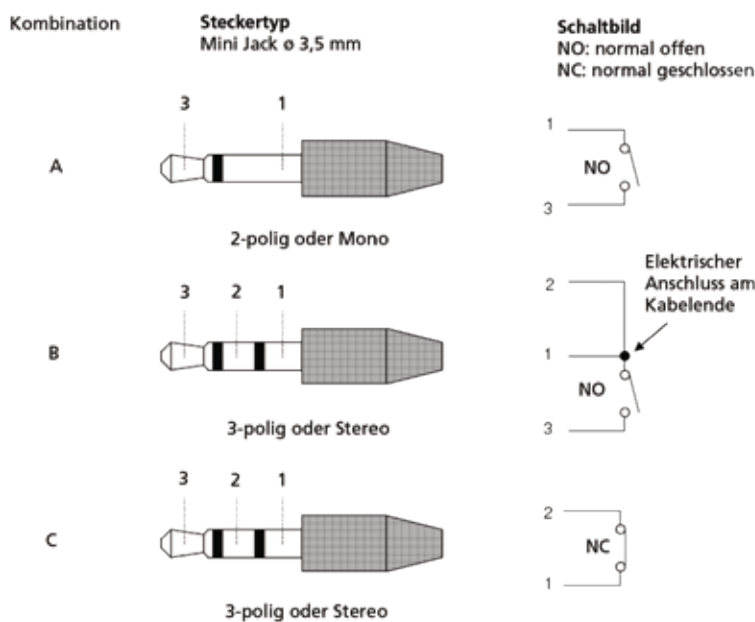
Abbildung 1: Kombinationen und entsprechende Schaltbilder sowie Funktionalitäten für den SLS
