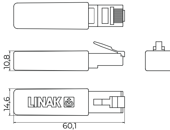
Abbildung 1 Bluetooth®-Adapter
