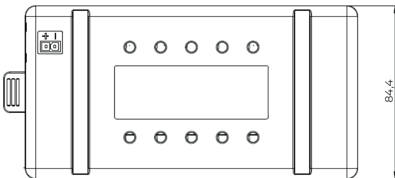
Abbildung 1 BA002 Abmessungen (mm)
