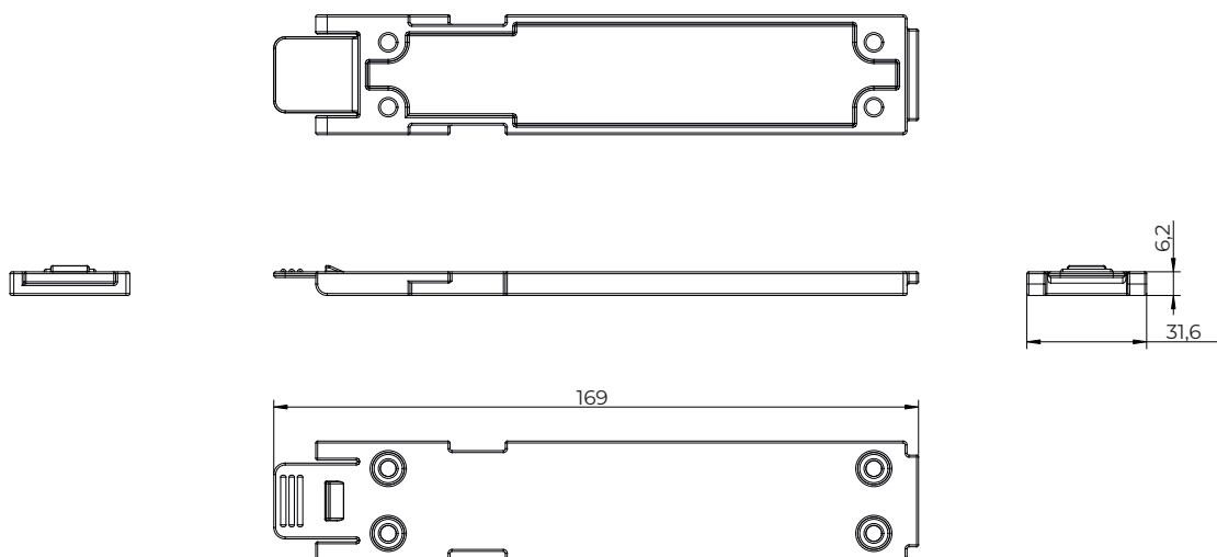
Abbildung 1 BA002 Abmessungen (mm)
