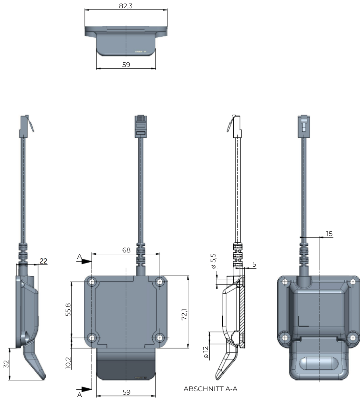
Abbildung 1 Maße DPIIK (mm)
