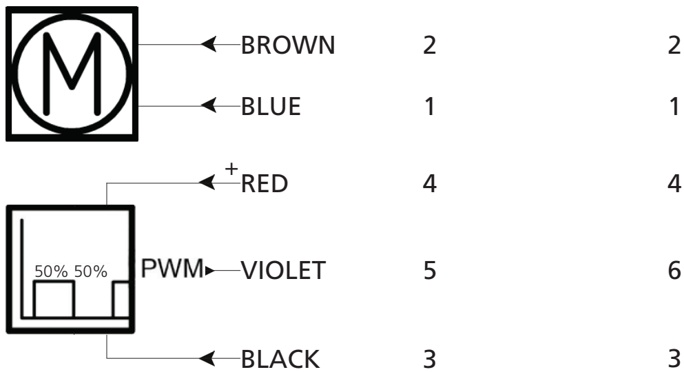
AMP 5P
